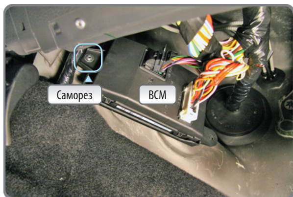
Фото 4. Блок ВСМ и его крепление
