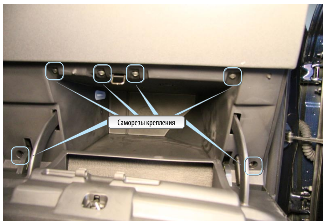
Фото 3.3. Крепление бардачка
