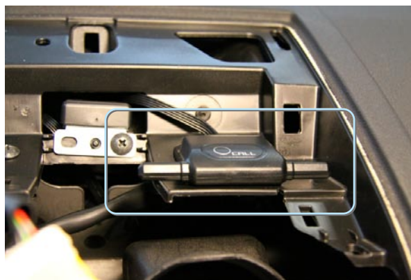
Фото 5.4. Антенна под облицовкой магнитолы
