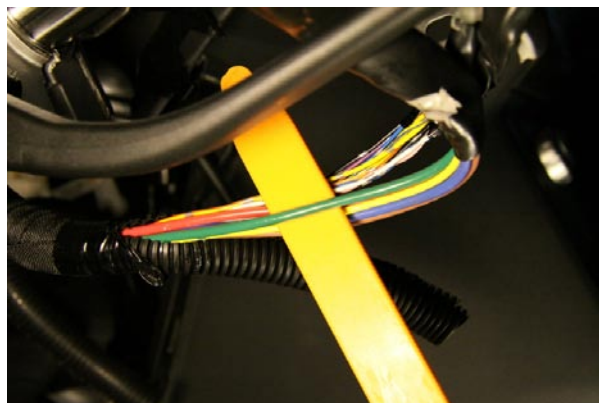
Фото 13.1. Зажигание IGN1 — зеленый
