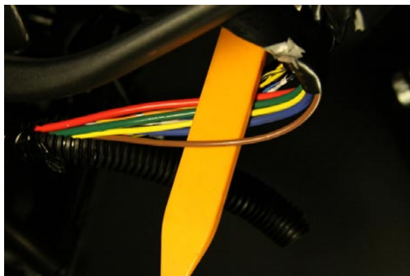
Фото 14. Аксессуары ACC — коричневый
