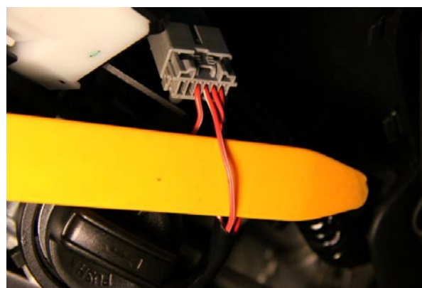
Фото 15.2. Провод питания-красный с белой полосой
