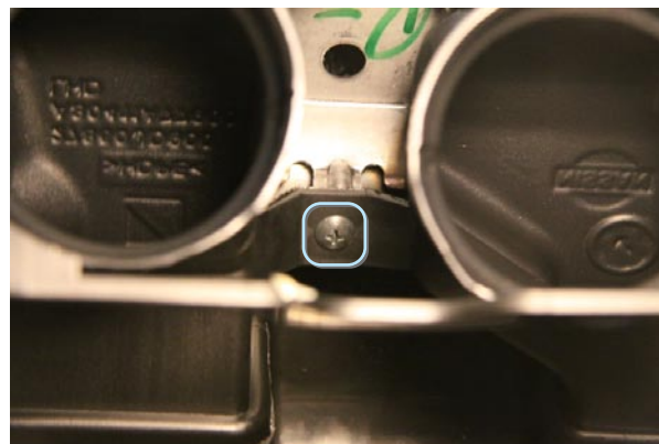
Фото 2.6. Крепление воздуховодов
