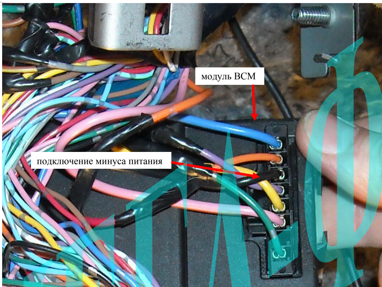
Рис. 12: Подключение минуса питания.
