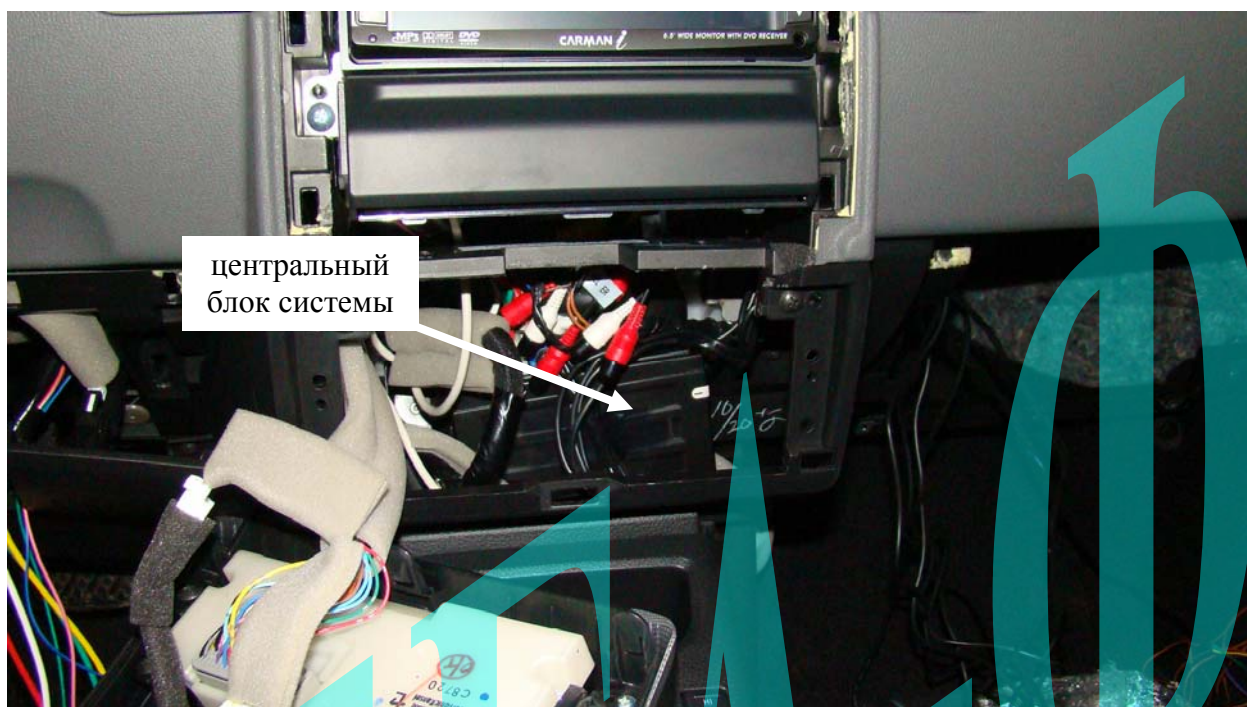
Рис. 11: Расположение центрального блока.
