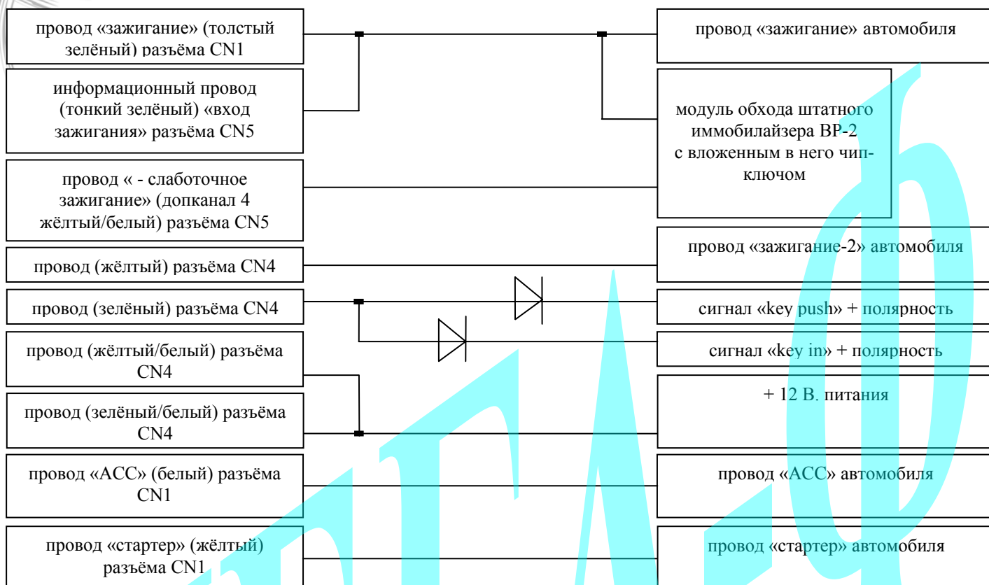
Схема 1: Подключение цепей запуска для автомобиля Nissan X-Trail комплектации ИК.
