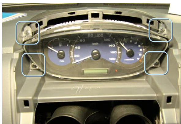
Фото 1.2. Крепление приборного щитка
