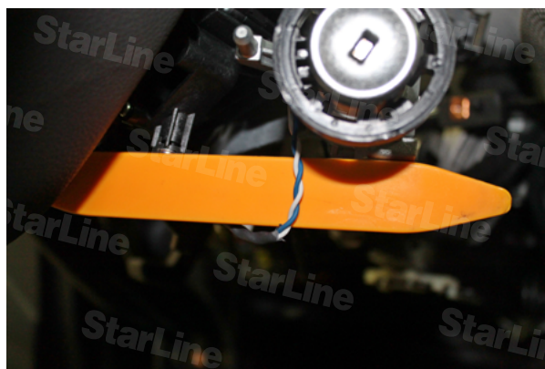
Фото 12. Провода рамки штатного иммобилайзера (белый и синий)
