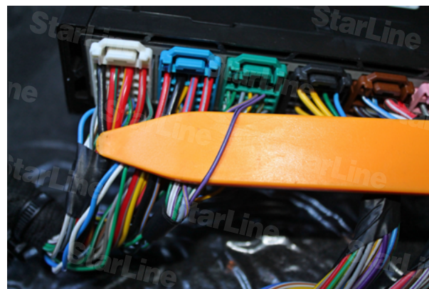
Фото 10.2. Зажигание (фиолетово-чёрный, pin 13)
