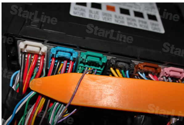
Фото 10.1. Аксессуары (фиолетово-жёлтый, pin 12)
