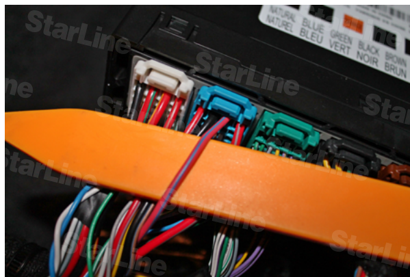
Фото 11. Питание +12В (красно-синий, pin 3)
