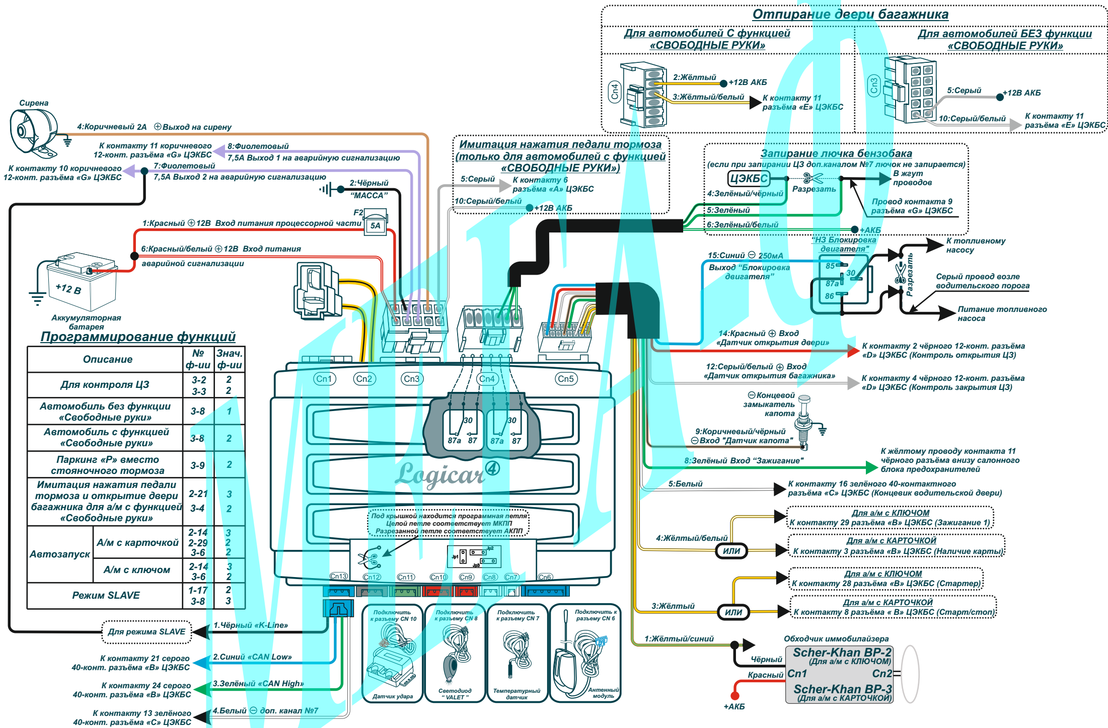
Схема подключения системы Scher-Khan Logicar 4 к автомобилю Renault FLUENCE
