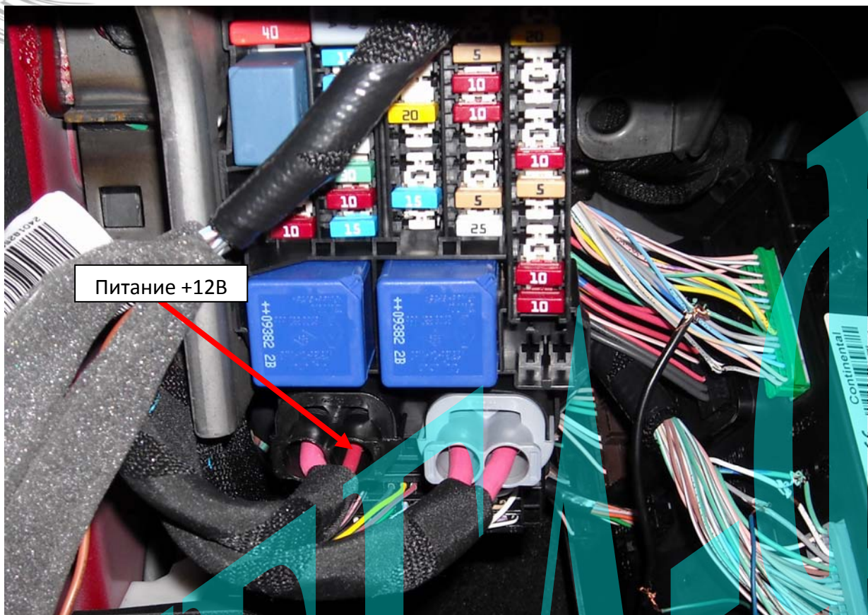
Рис. 17: Подключение питания.
