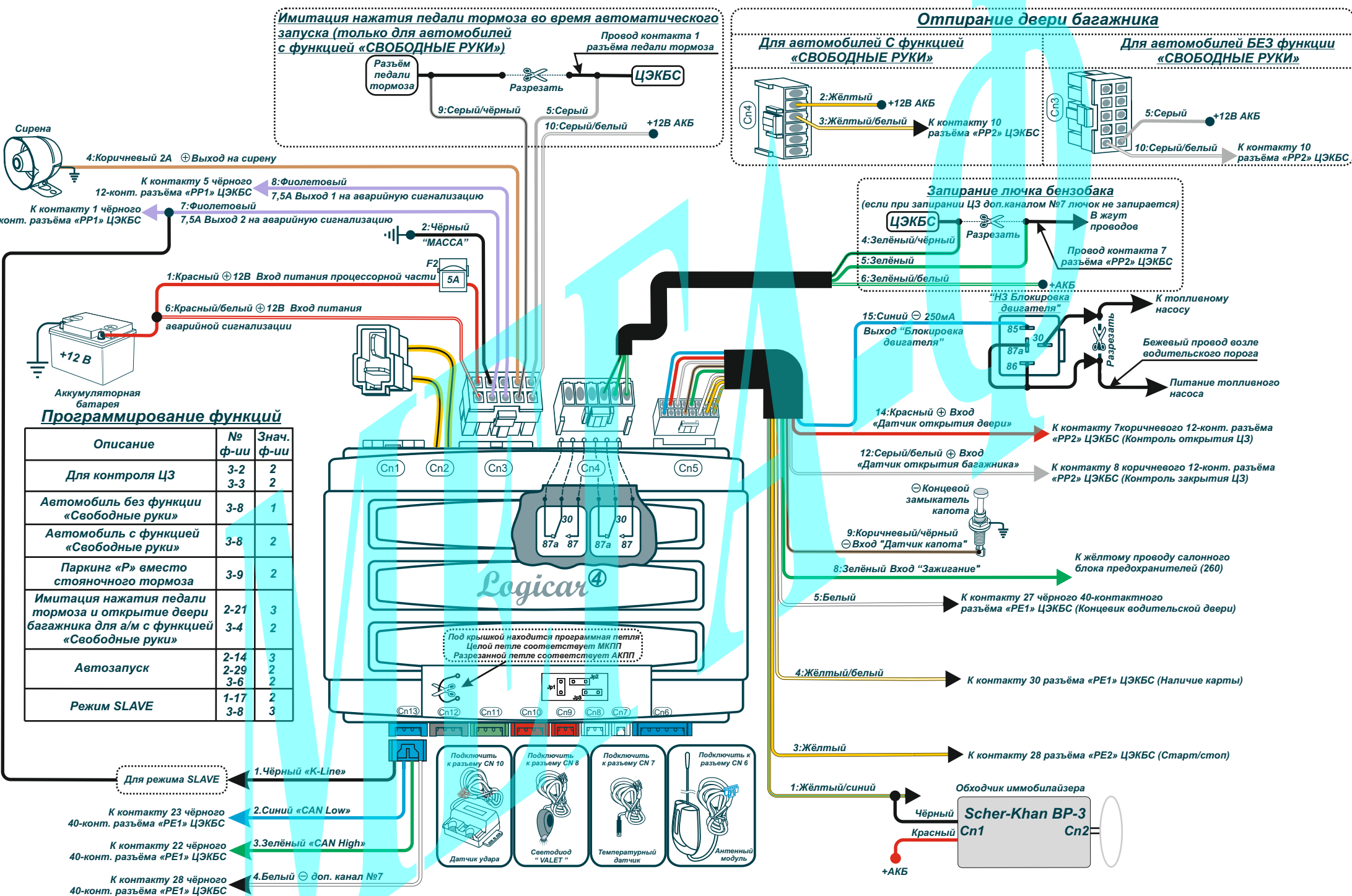
Схема подключения системы Scher-Khan Logicar 4 к автомобилю Renault LATITUDE
