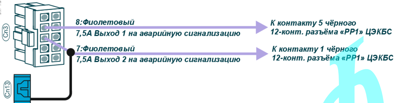
Схема 11: Подключения, необходимые для режима «Slave».
