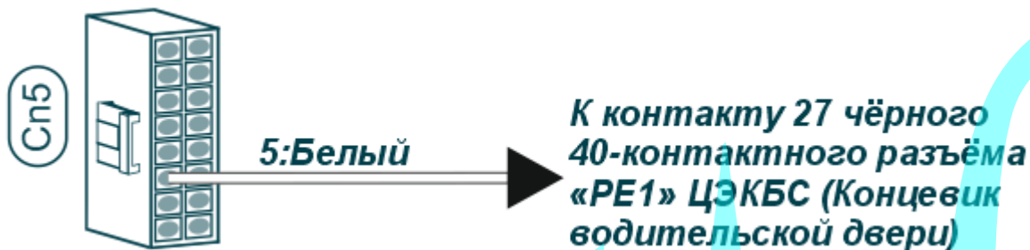
Схема. 6: Подключение имитации открытия водительской двери.
