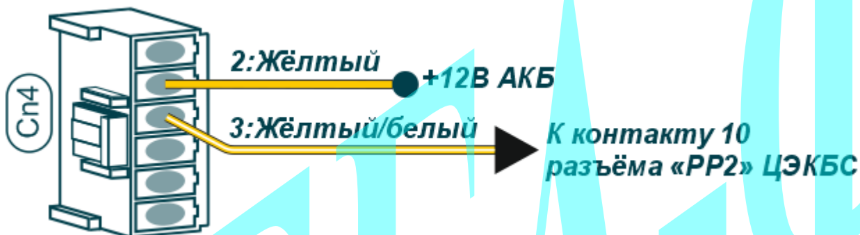
Схема 9: Подключение цепи управления замком багажника на автомобилях с функцией «Свободные руки».
