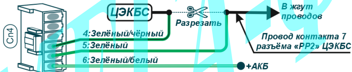
Схема 3: Подключение замка лючка бензобака.
