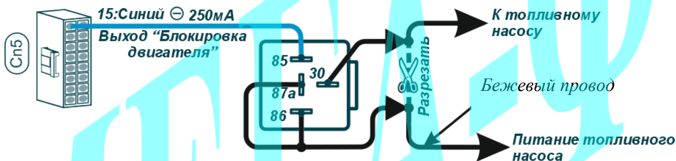
Схема. 8: Подключение цепи блокировки.
