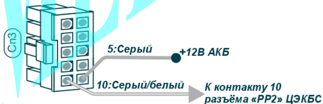
Схема 10: Подключение цепи управления замком багажника на автомобилях без функции «Свободные руки».
